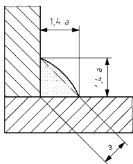
Εικόνα 1.3 Διαστάσεις εξωρραφών
