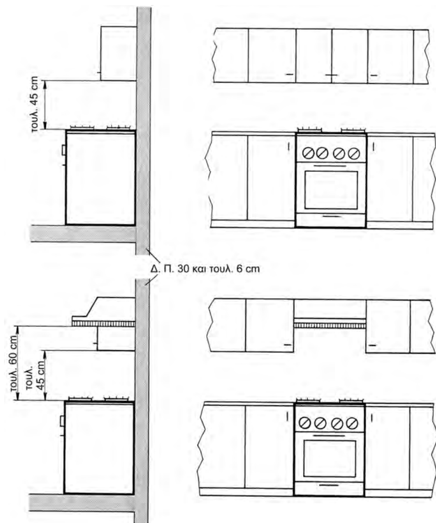
Εικόνα 8.2 Παράδειγμα εγκατάστασης μαγειρικών εστιών (ελεύθερη ή εντοιχισμένη)
