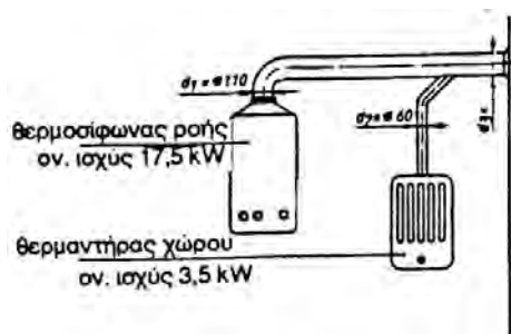
Εικόνα 9.2 Σύνδεση με κοινό καπναγωγό θερμαντήρα νερού και θερμαντήρα χώρου
