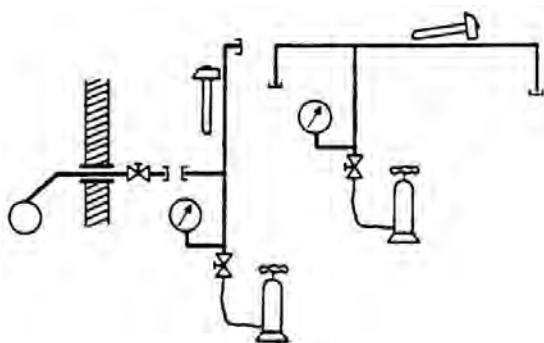
Εικόνα 10.1 Δοκιμή αντοχής
